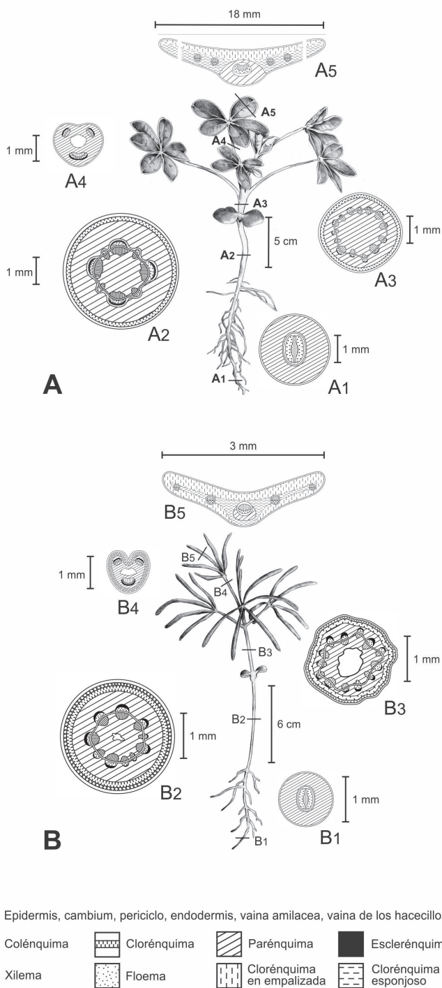
Fig. 1. Representación del estado de crecimiento promedio de las plántulas de L. albus (A) y L. angustifolius (B) a los 20 días después de la siembra y diagramas tisulares de las secciones transversales de los órganos según los patrones de Metcalfe & Chalk [1950], más esquemas especiales diseñados para el trabajo. A1, B1: Raíz primaria; A2, B2: Hipocótilo. A3, B3: Epicótilo. A4, B4: Pecíolo. A5, B5: Folíolo.
