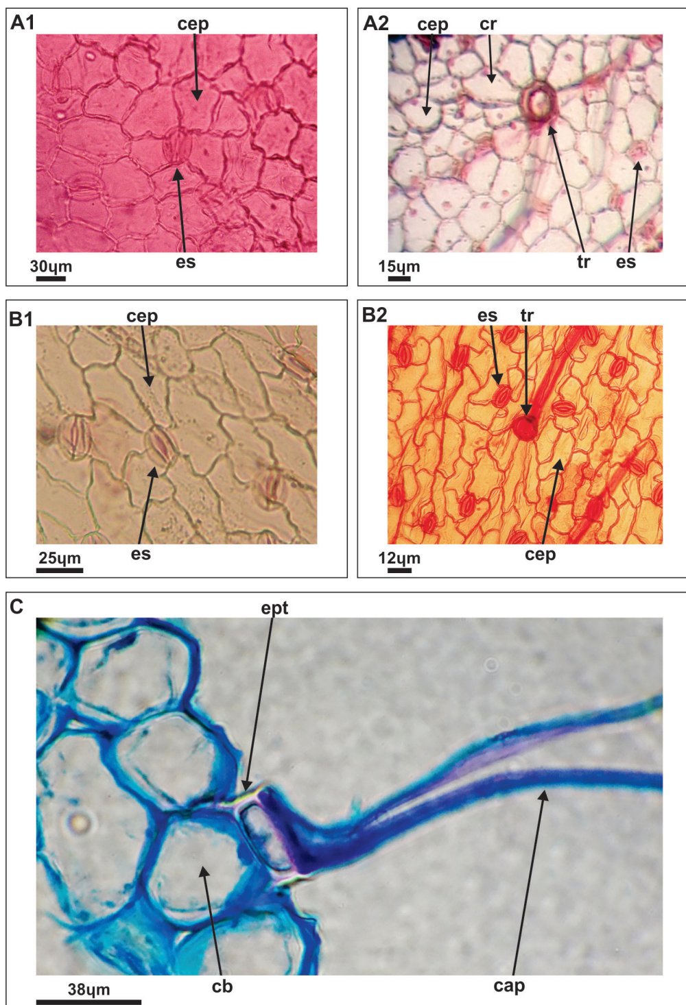
Fig. 4. Fotomicrografías de epidermis en vista superficial. A) L. albus . B) L. angustifolius . A1, B1: Epidermis adaxial. A2, B2: Epidermis abaxial. Referencias: cep, célula epidérmica; es, estoma; cr células radiales. C) Corte transversal del folíolo mostrando la epidermis y un tricoma tricelular. Referencias: cap, célula apical; cb célula basal; ept, epitricopodium.
